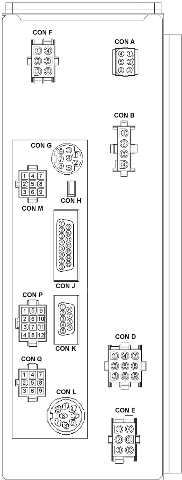
[ 制御盤背面 ]
