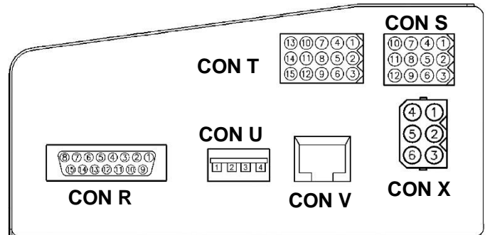
[ ミシン頭部背面 / F ユニット ]
